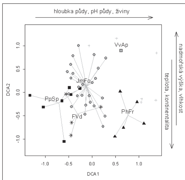
Obr. 3. Ordinační diagram detrendované korespondenční analýzy (DCA). Fytoecologické snímky klasifikované do stejné asociace jsou spojeny šedou čarou s těžištěm každé skupiny (pavoučí diagram) a toto těžiště je označeno zkratkou odpovídající asociace. Šipky na horní, respektive pravé straně diagramu znázorňují směr korelace vybraných proměnných prostředí s první, respektive druhou ordinační osou. Neklasifikované snímky jsou zobrazeny šedými křížky.
